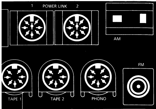
Beomaster 7000
